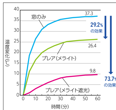
夏の室内温度推移
