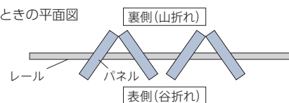
パネルを折ったときの平面図
